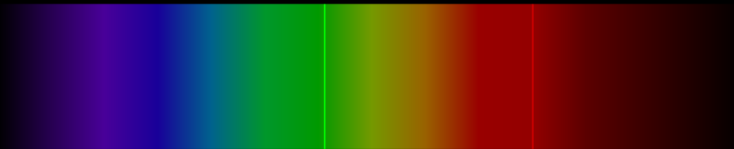
K_5
