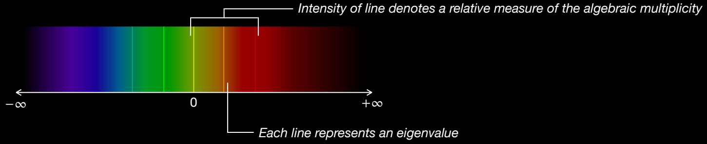
K_5
